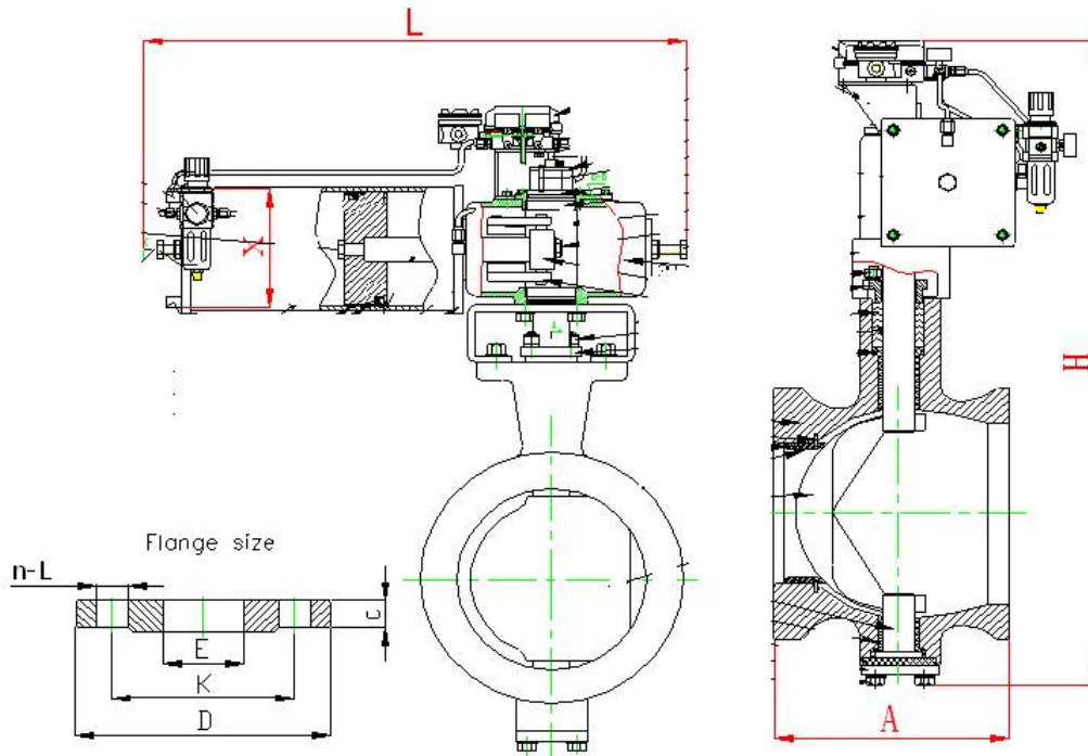
V 型球閥外型主要尺寸 (mm) (單動致動器&對夾式連接)
