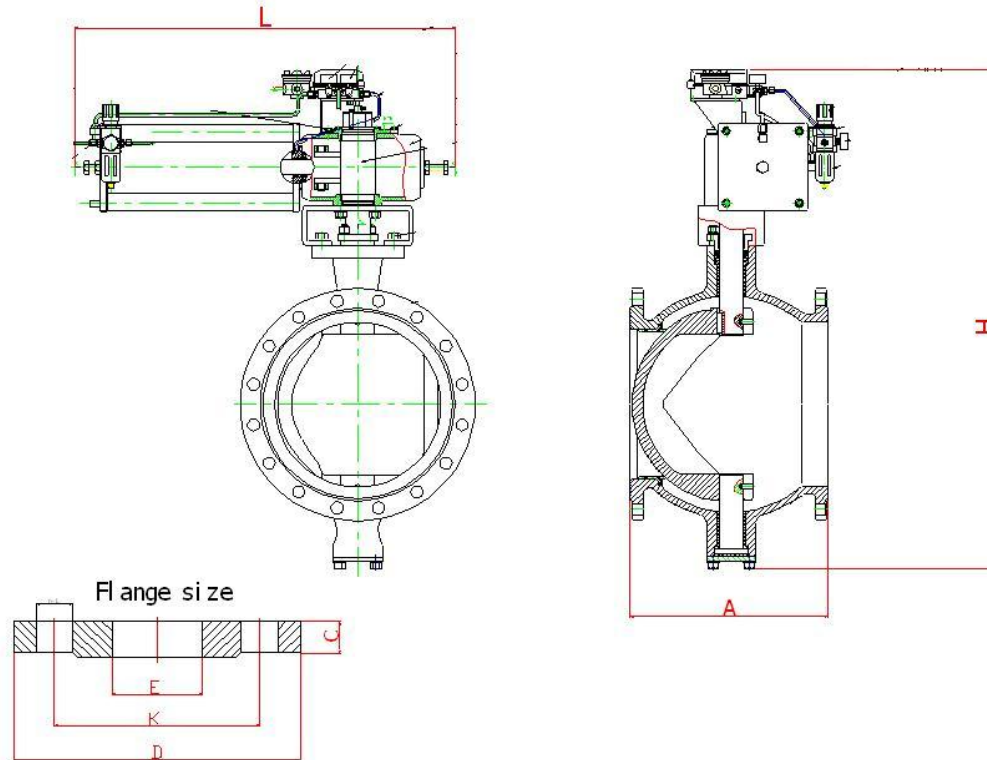
V 型球閥外型主要尺寸 (mm) (單動致動器&法蘭式連接)
