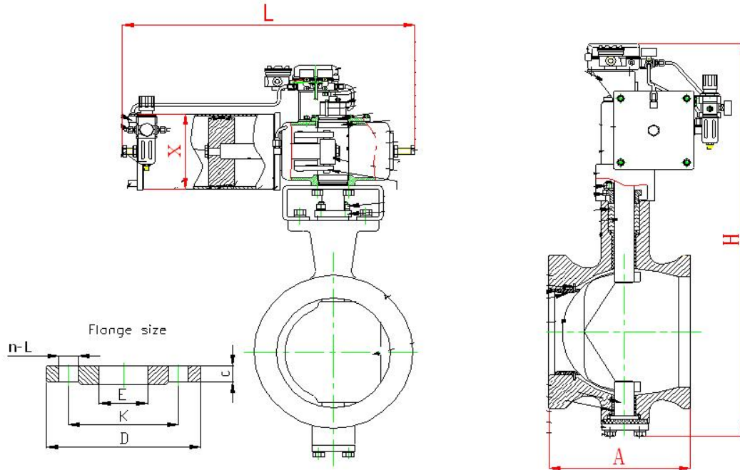
V 型球閥外型主要尺寸 (mm) (雙動致動器&對夾式連接)
